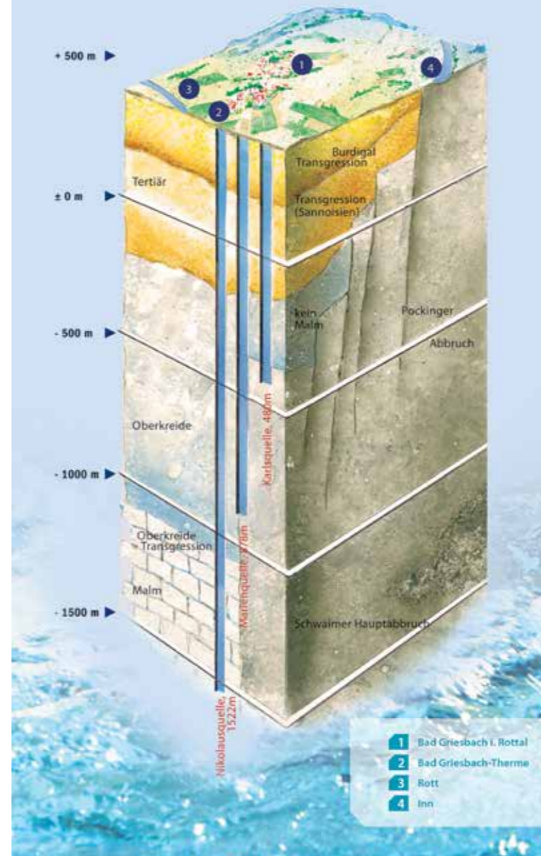
Geologisches Blockbild der Thermalwasserquellen „Nikolausquelle“, „Marienquelle“ und „Karlsquelle“
